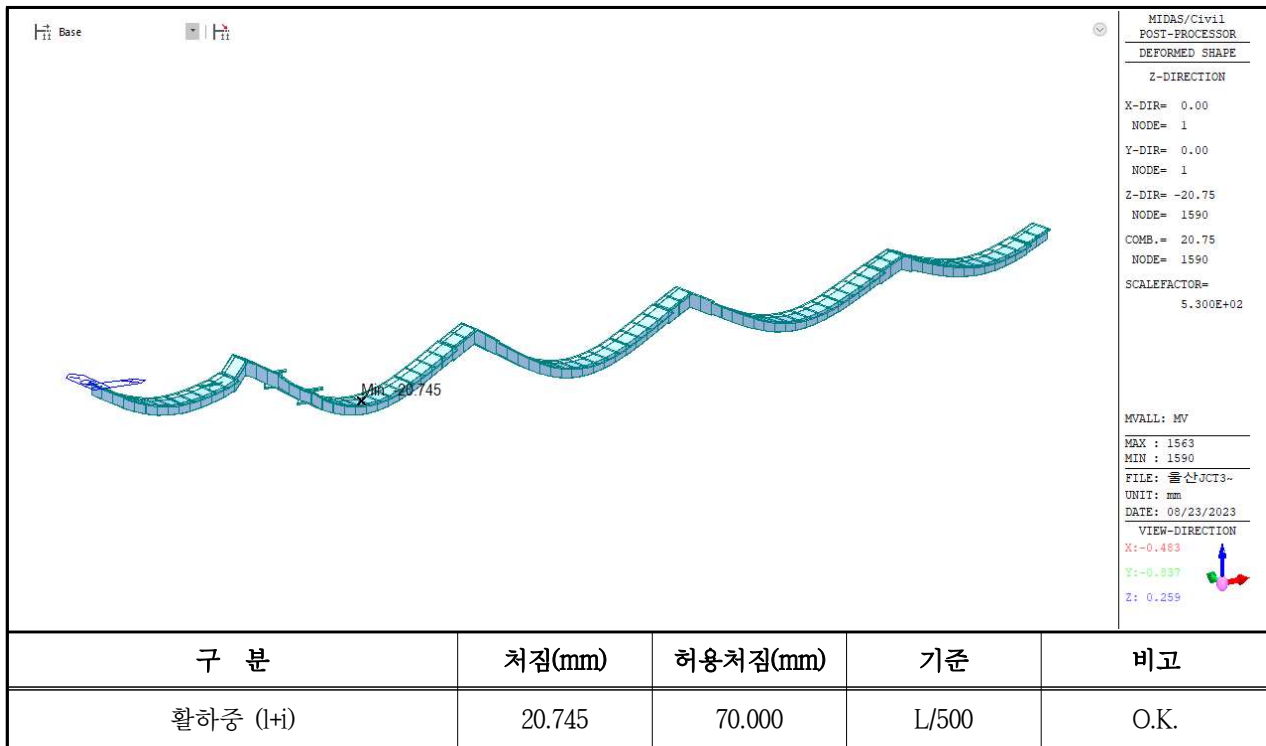
【그림 5.14】 처짐검토 결과
