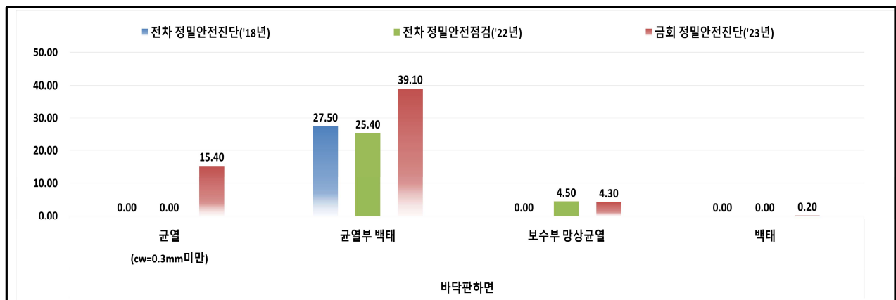
【그림 3.1】 바닥판 하면 기 진단 결과와의 비교
