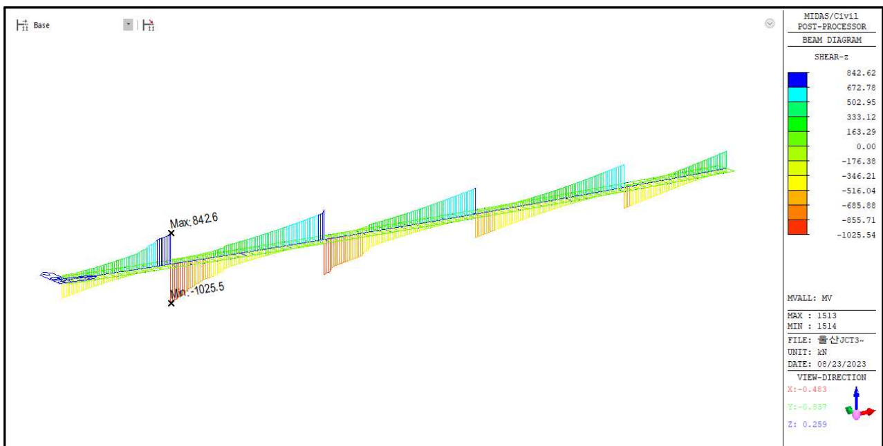
【그림 5.13】 활하중에 의한 전단력도
