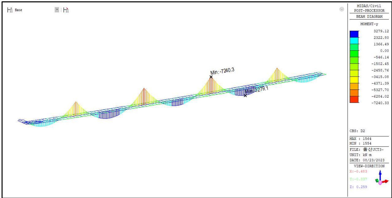
【그림 5.10】 합성후 고정하중에 의한 휨모멘트도
