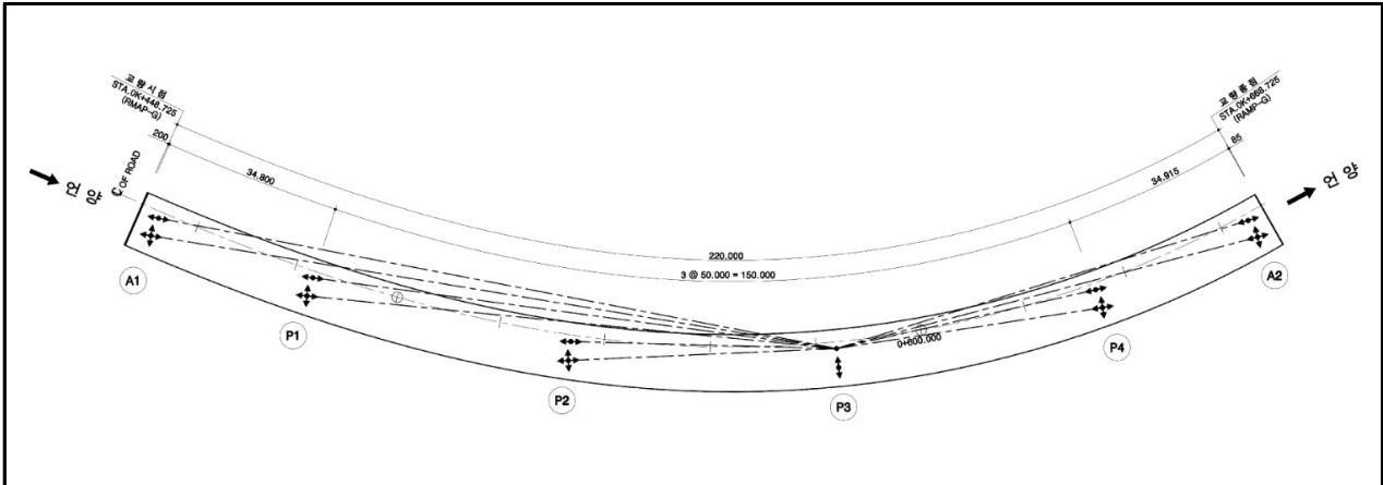
【그림 5.15】 받침배치도
