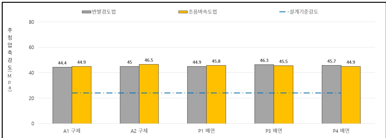
【그림 3.23】하부구조 추정비파괴강도 결과 그래프
