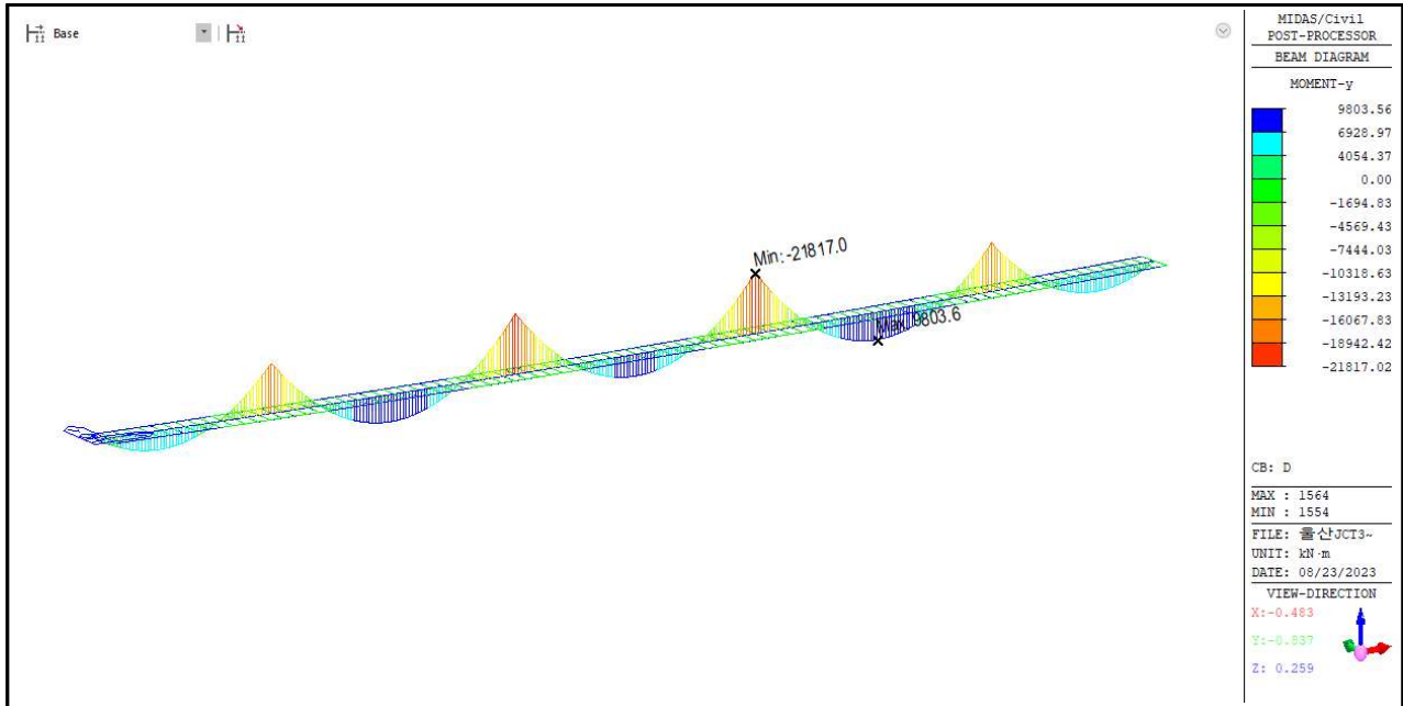
【그림 5.8】 합성전 고정하중에 의한 휨모멘트도
