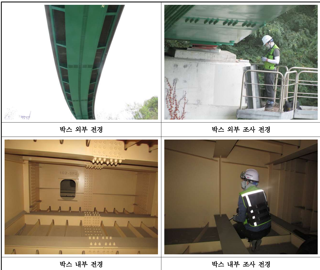
【사진 3.6】 강박스 거더 전경
