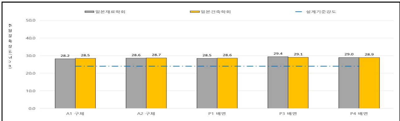
【그림 3.18】하부구조 반발경도 시험결과
