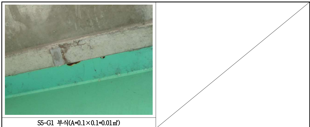
【사진 3.8】 강박스 거더 외부 손상현황
