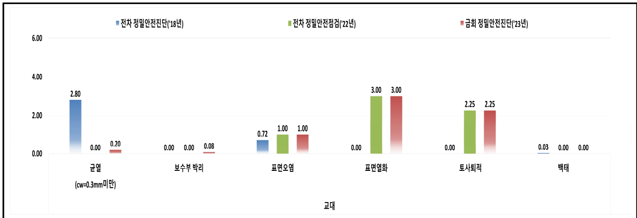
【그림 3.6】 교대 기 점검 결과와의 비교
