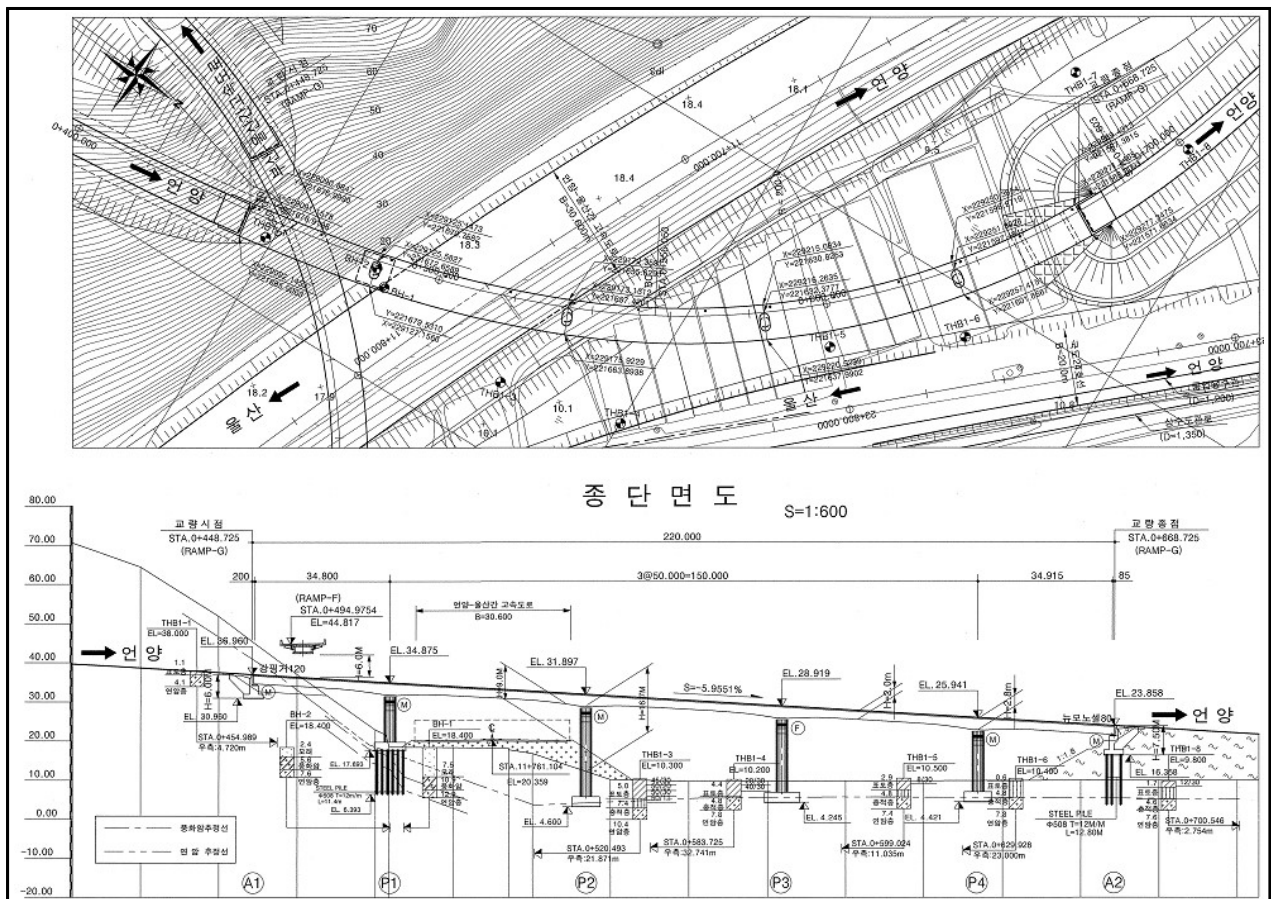
【그림 5.1】 종·평면도
