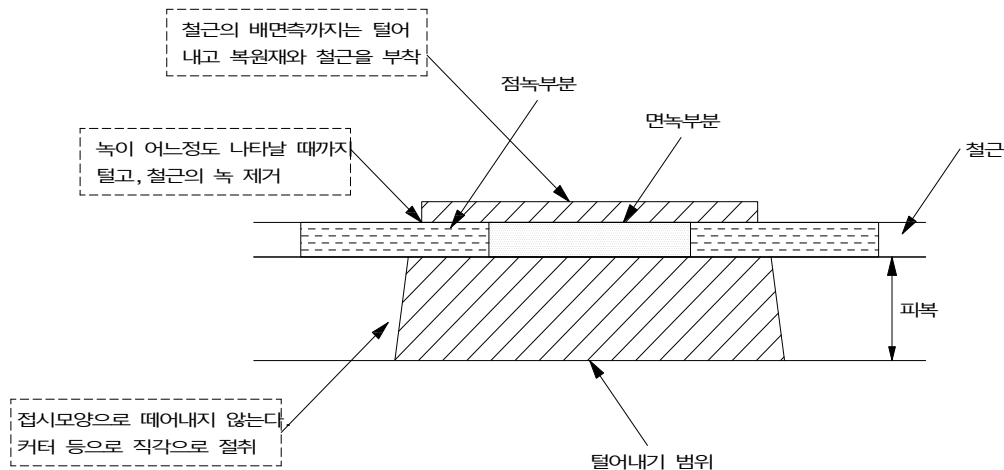
【그림 7.3】 단면복구(보수) 상세도
