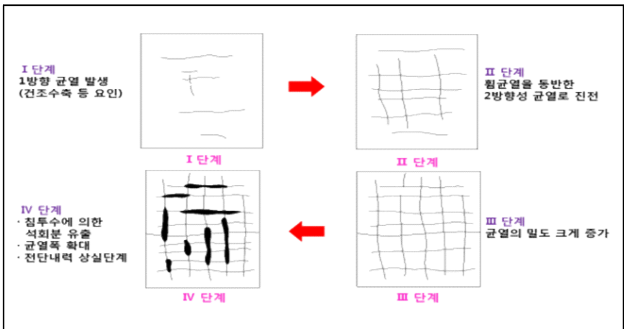
【그림 3.2】 콘크리트 바닥판의 균열진전 개요도
