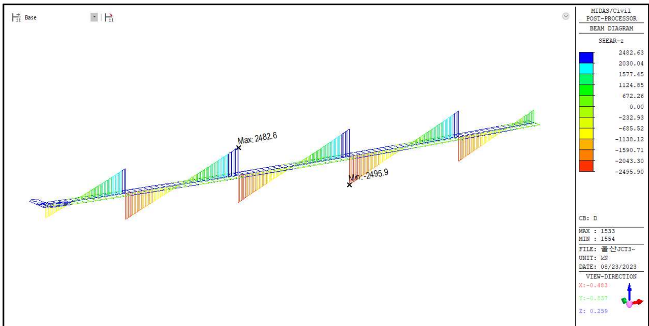
【그림 5.9】 합성전 고정하중에 의한 전단력도
