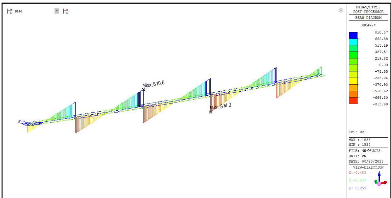
【그림 5.11】 합성후 고정하중에 의한 전단력도
