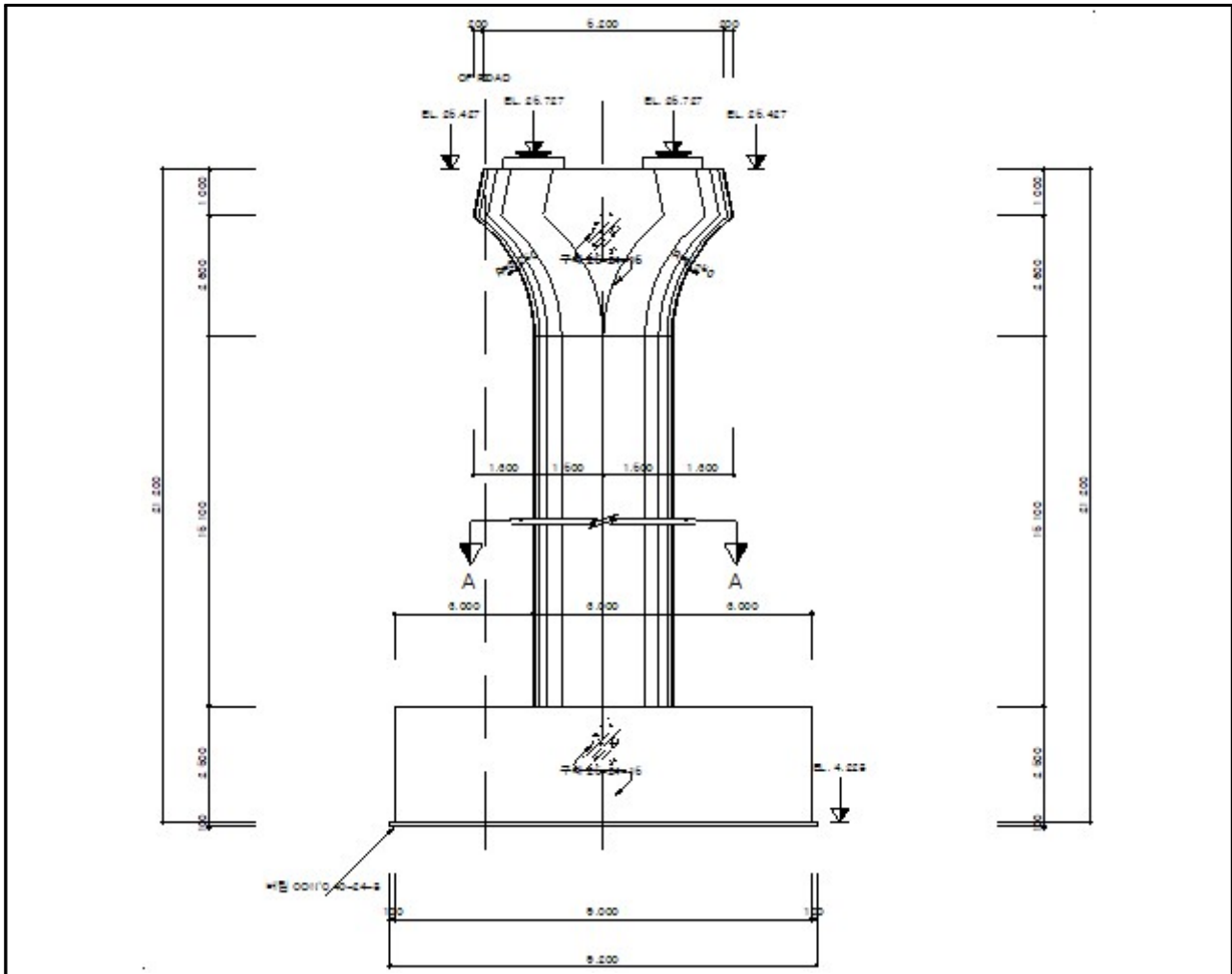
【그림 5.17】 해석단면(P3)
