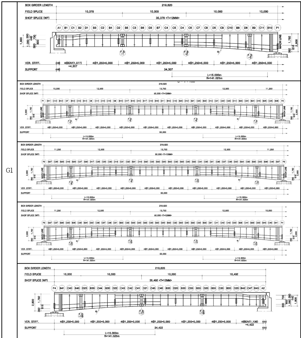
【그림 5.3】 단면배치도
