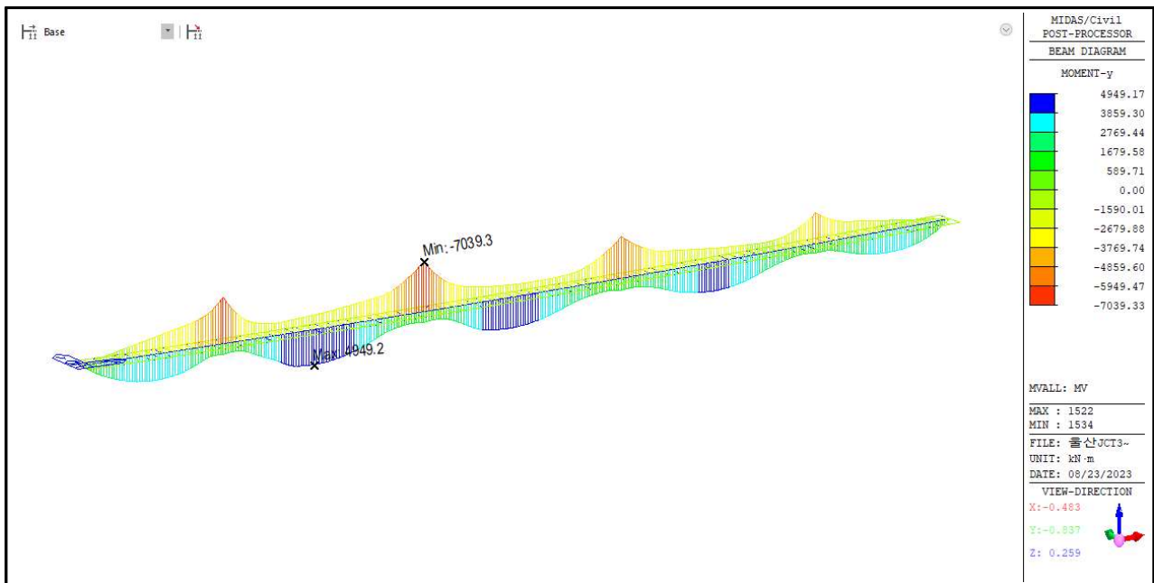
【그림 5.12】 활하중에 의한 휨모멘트도
