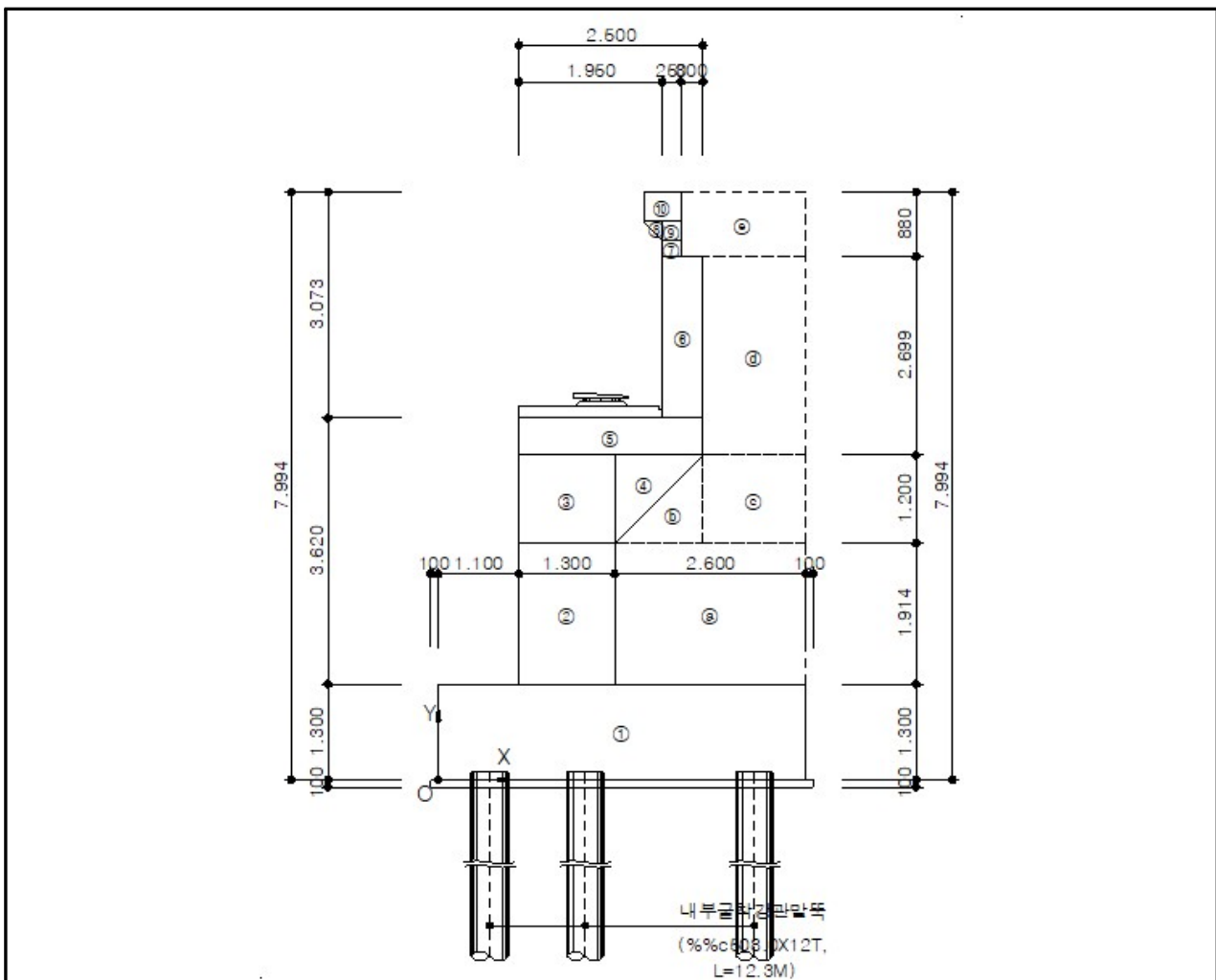
【그림 5.16】 해석단면(A2)
