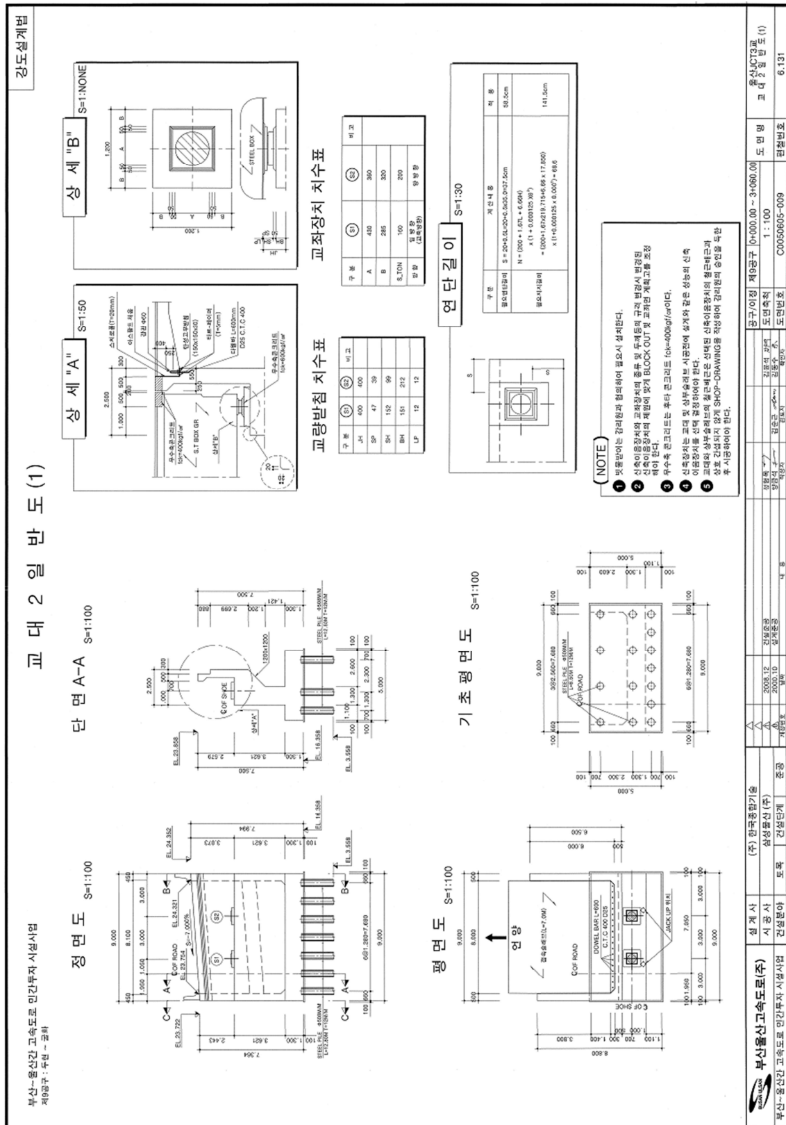
【그림 1.6】 교대 A2 일반도
