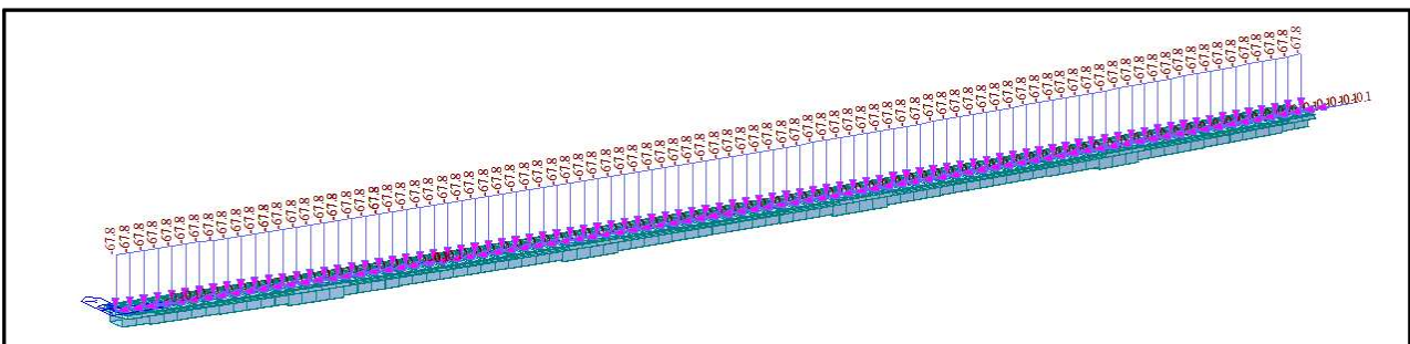
【그림 5.4】 합성전 고정하중(바닥판 하중) 재하도
