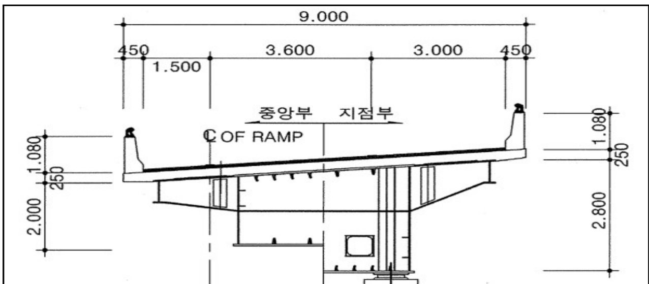
【그림 5.2】 횡단면도
