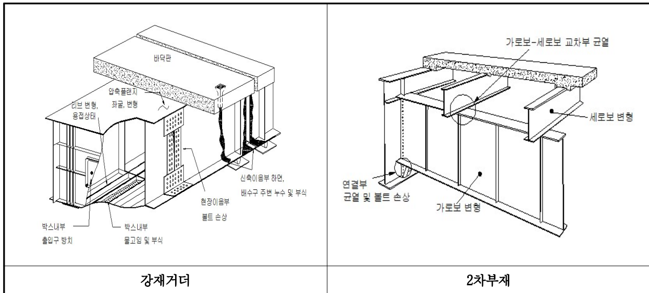
【그림 3.3】 강박스 거더의 일반적인 손상
