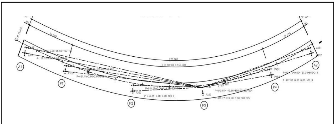
【그림 3.8】 교량받침 배치도
