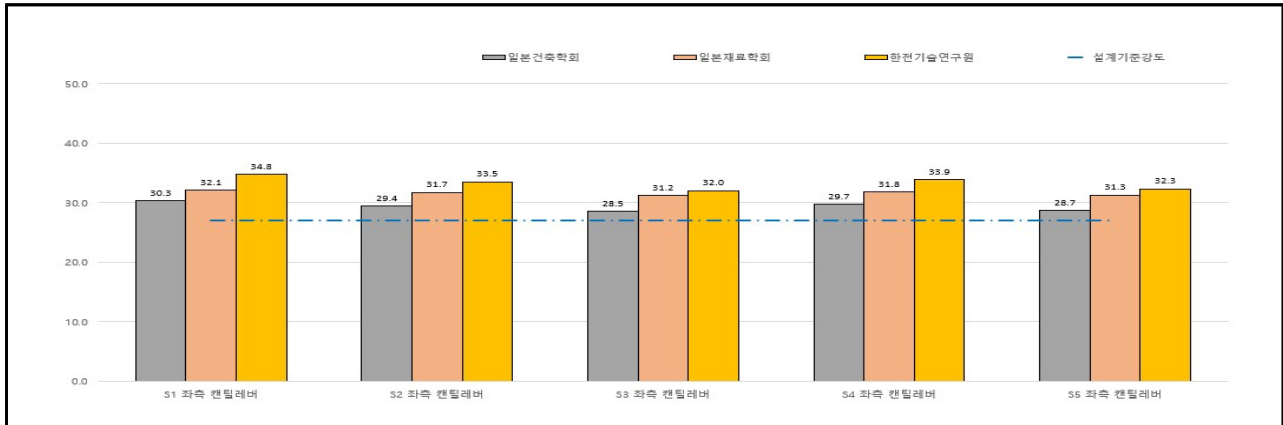
【그림 3.20】 상부구조 초음파 전달속도 시험결과
