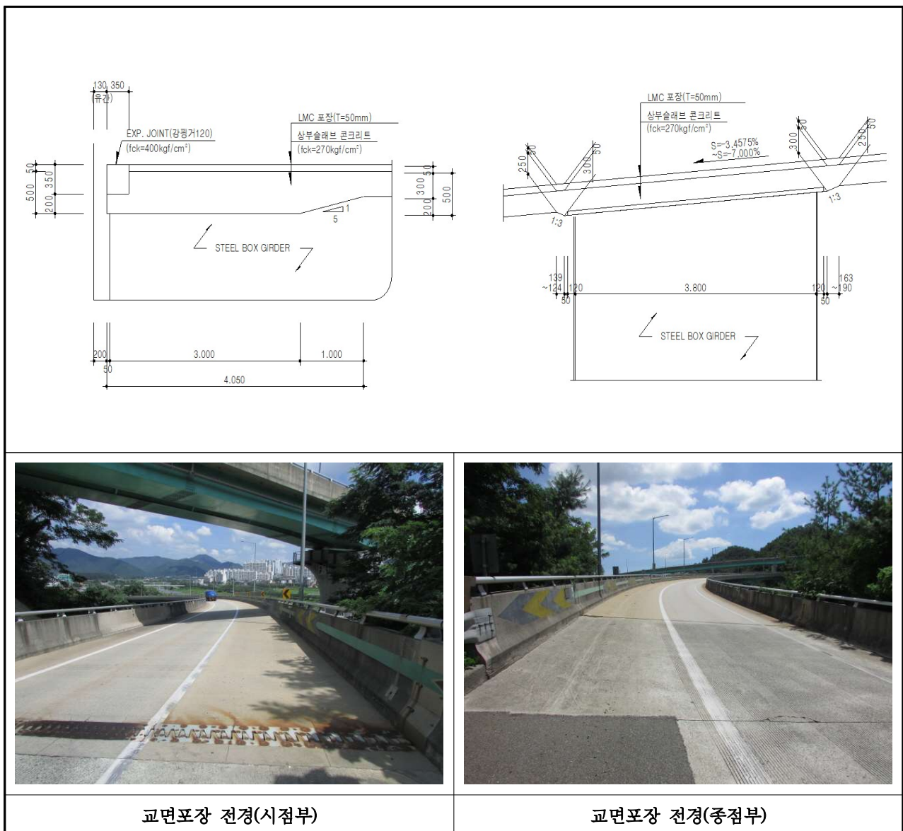
【사진 3.21】 교면포장 전경 및 상세도
