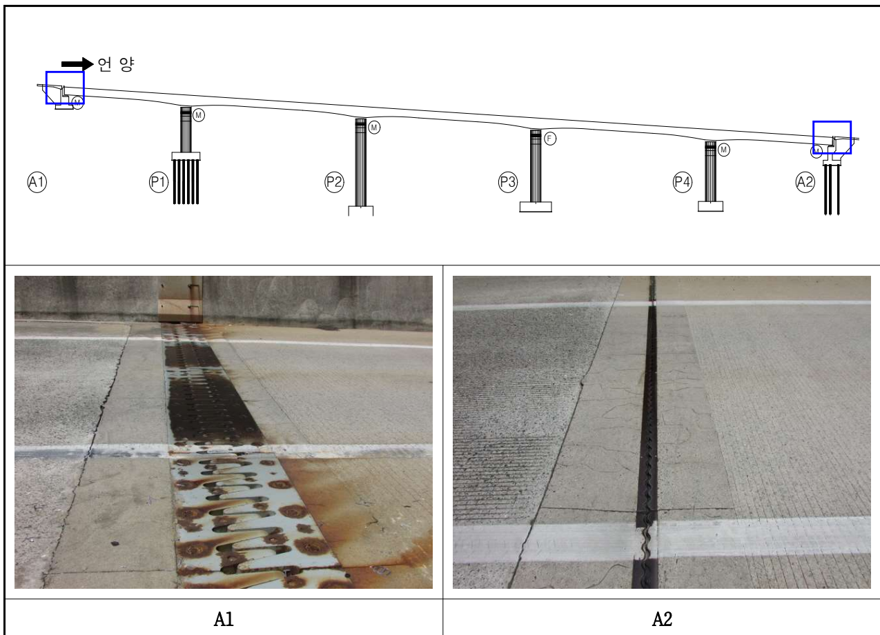
【그림 3.11】 신축이음장치 전경 및 배치도
