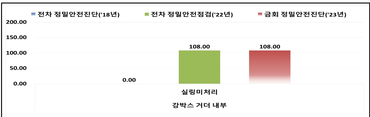
【그림 3.4】 거더 내부 기 진단 결과와의 비교
