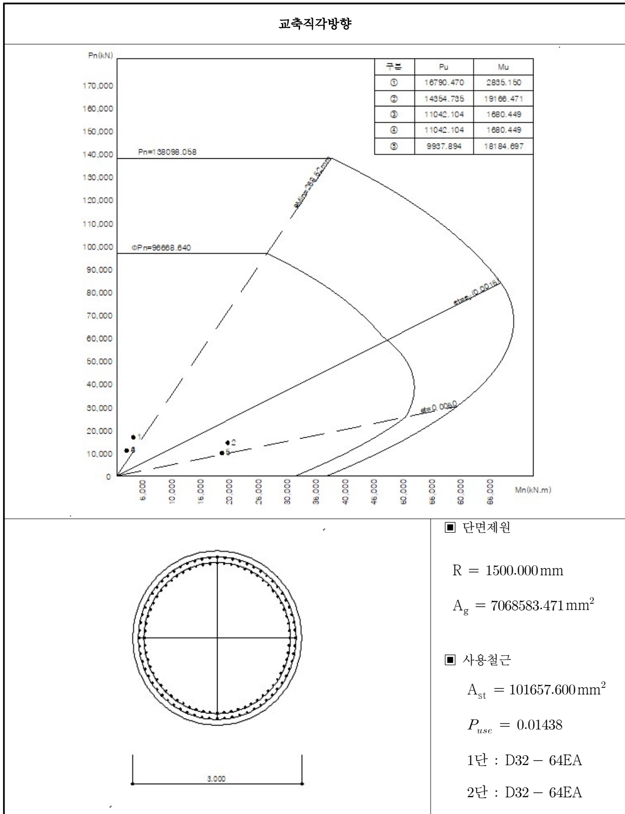
【그림 5.19】 교축직각방향 P-M상관도(P3)
