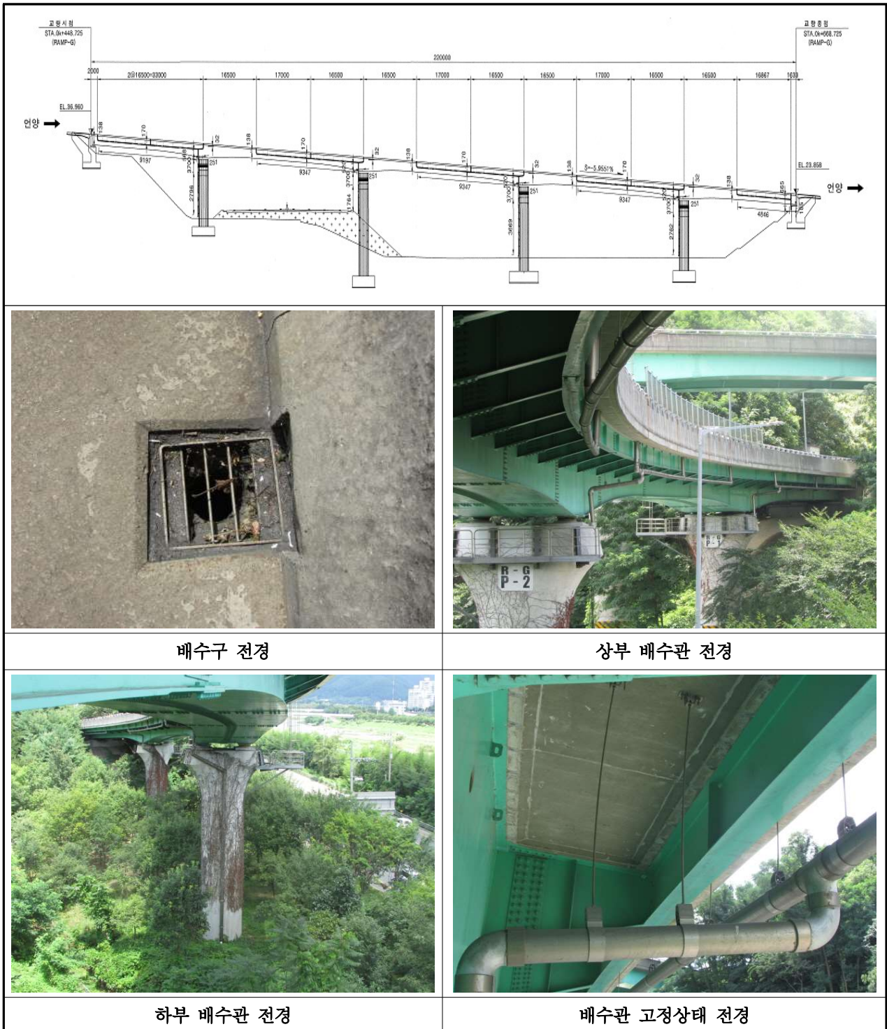
【사진 3.23】 배수시설 위치도 및 전경
