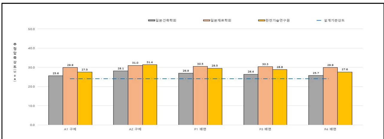
【그림 3.21】 하부구조 초음파 전달속도 시험결과
