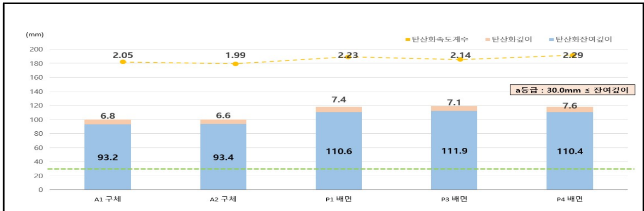
【그림 3.26】하부구조 탄산화 깊이 측정 결과
