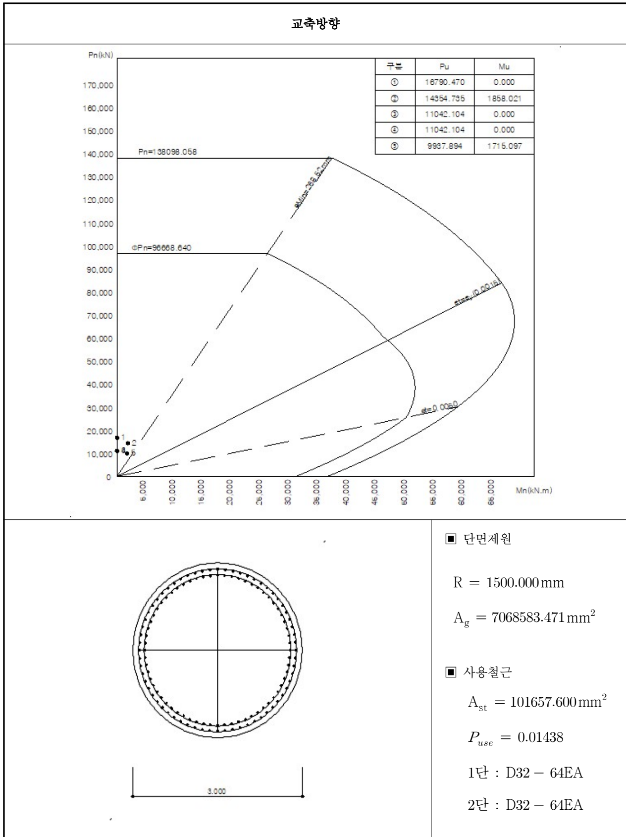
【그림 5.20】 교축방향 P-M상관도(P3)
