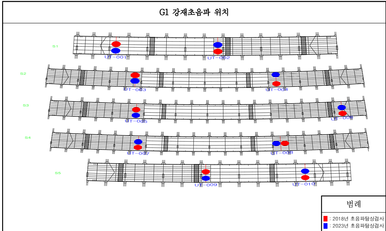
【그림 3.28】 강재 초음파 탐상시험(U.T) 위치도
