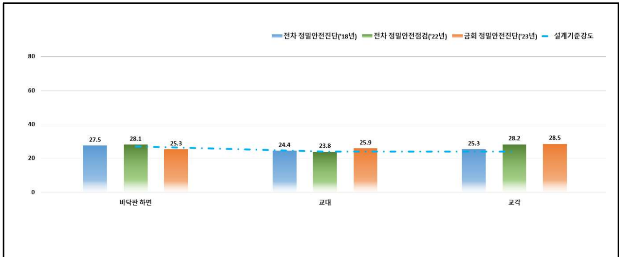
【그림 3.19】 전차 정밀안전진단 및 전차 정밀안전점검 결과 비교
