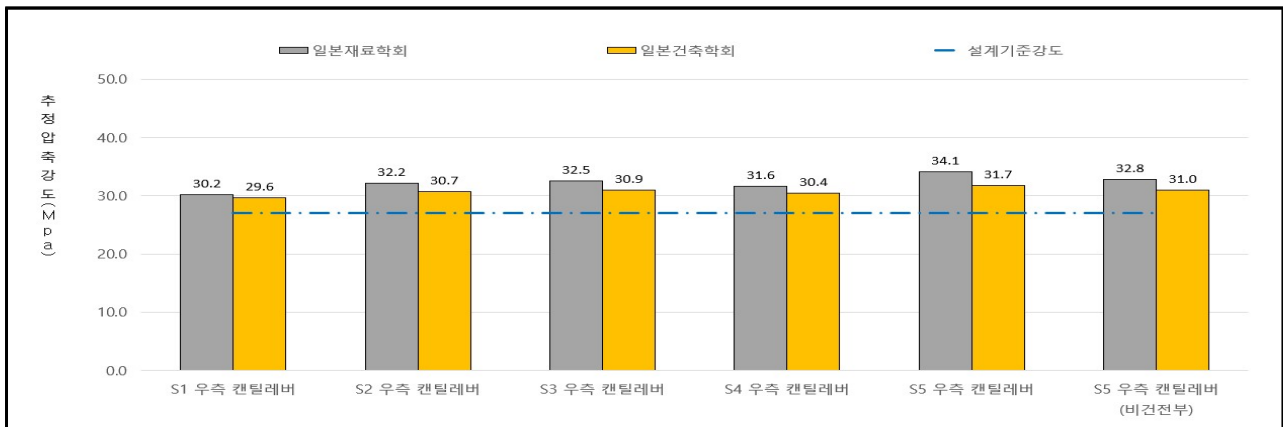
【그림 3.17】 상부구조 반발경도 시험결과
