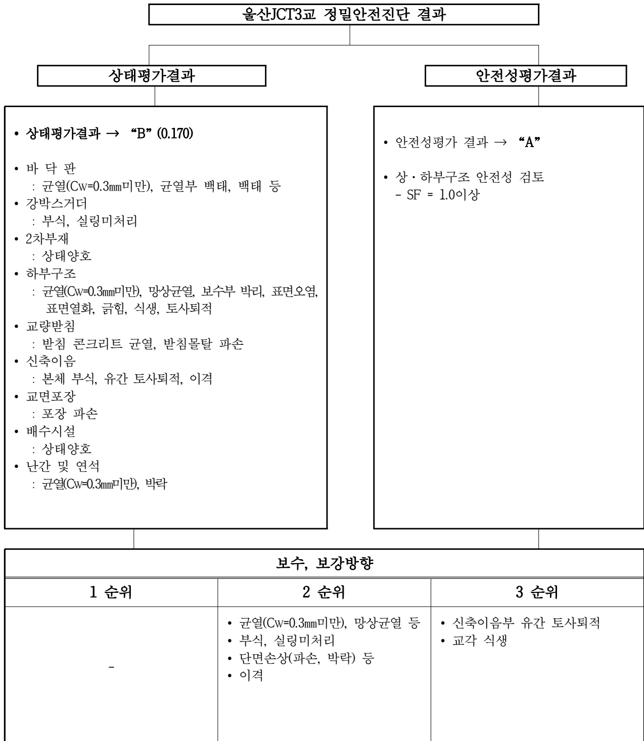
【그림 7.1】 보수·보강방안 추진방향
